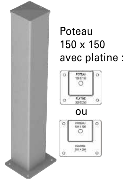
Poteau 150 x 150 à sceller
