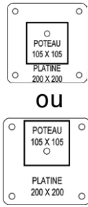
Poteau 105 x 105 sur platine
