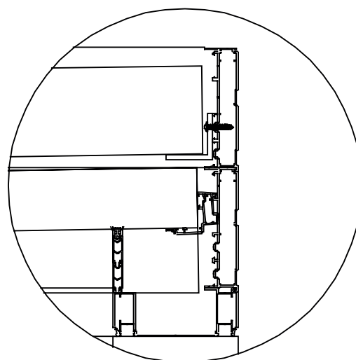
Détail fixation haute
