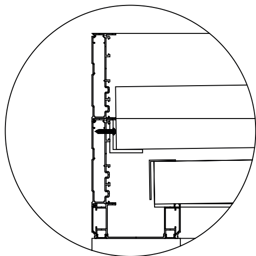
Détail fixation basse
