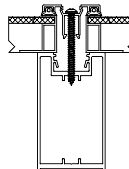
Détail fixation panneaux
