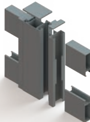
Détail poteau avec montant de dilatation
